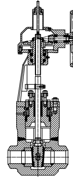
Управление через редуктор
