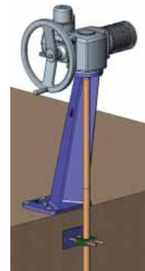
Наклонная колонна
